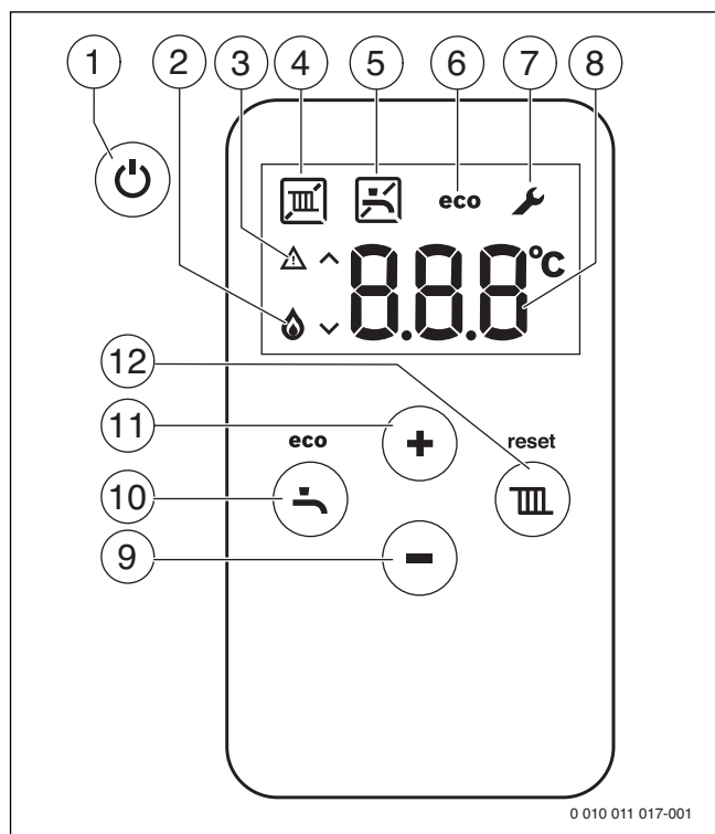
Fig. 6 Afișaje pe ecran
